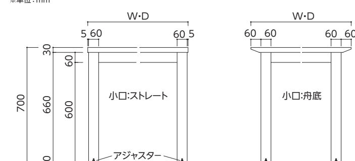
脚のみの高さはH690まで対応できます
